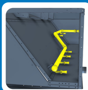
Патрубки очистки поддона
